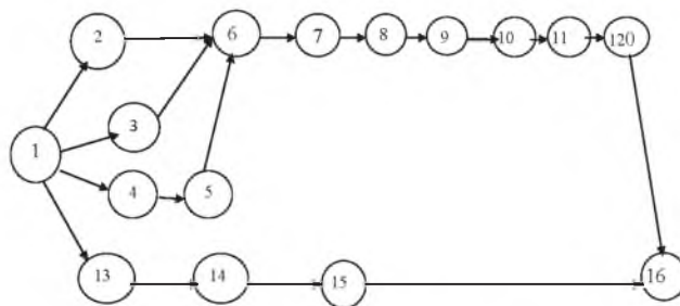
Рис. 2. Сіткова модель
