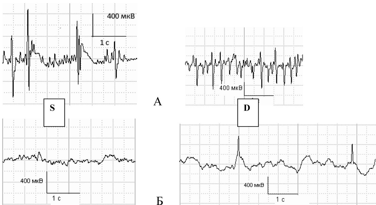
Рис. 2. S – ліва півкуля, D – права півкуля. A – ЕКОГ при моделюванні вогнищевої епілепсії, Б – ЕКОГ при моделюванні вогнищевої епілепсії на фоні дії вальпроату натрію
