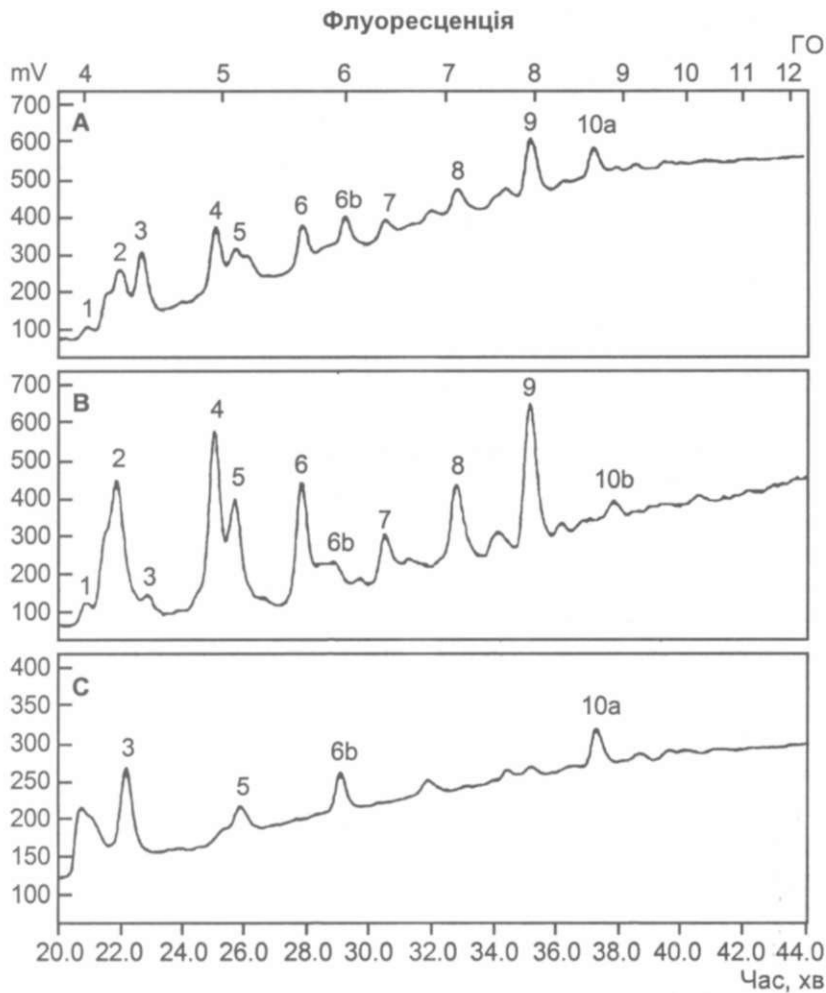
Рис. 2. Порівняння ВЕРХ-спектрів загального пулу (А), нейтральної (В) і зарядженої (С) фракцій вільних олігосахаридів плазми крові хворих на хронічну серцеву недостатність і практично здорових донорів (плазма хворого до лікування)
