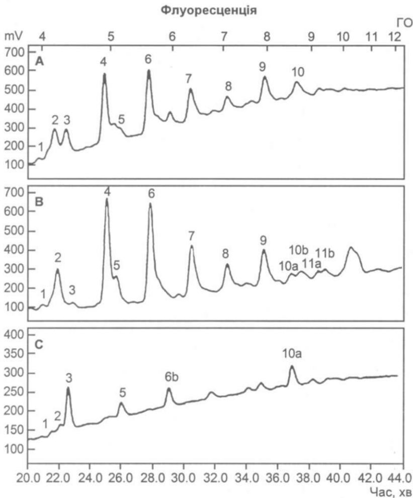
Рис. 3. Порівняння ВЕРХ-спектрів загального пулу (А), нейтральної (В) і зарядженої (С) фракцій вільних oligосахаридів плазми крові хворих на хронічну серцеву недостатність і практично здорових донорів (плазма хворого після лікування)
