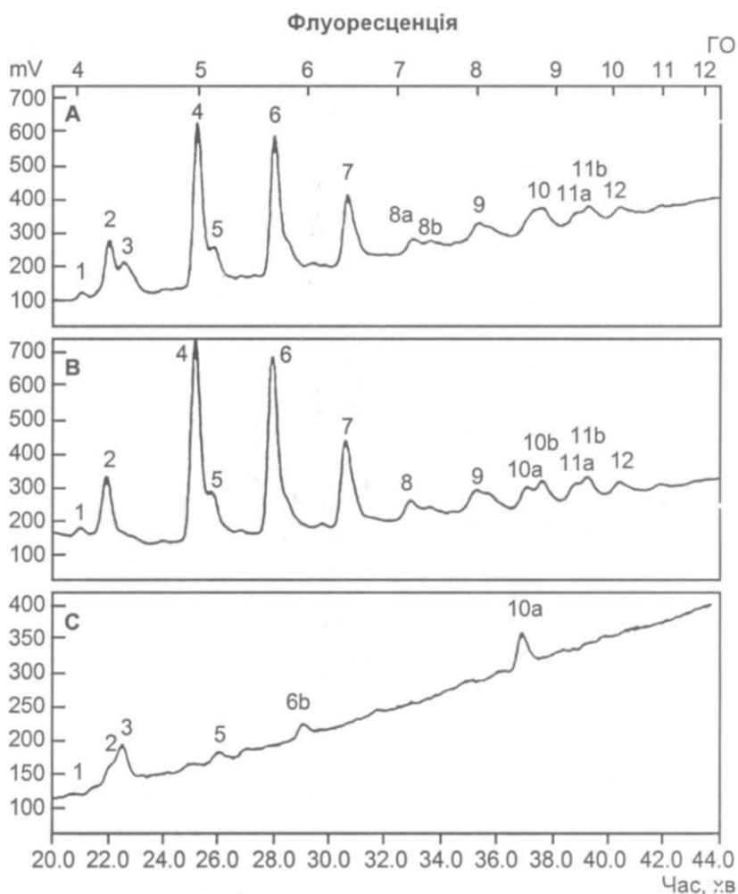
Рис. 1. Порівняння ВЕРХ-спектрів загального пулу (А), нейтральної (В) і зарядженої (С) фракцій вільних олігосахаридів плазми крові хворих на хронічну серцеву недостатність і практично здорових донорів (контроль)
