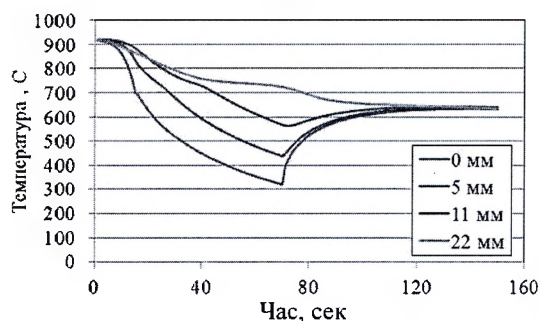
Рис. 2. Зміна температури по перетину головки рейки в процесі термічної обробки (гартування і самовідпуску)/
